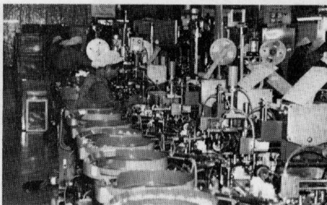
冷蔵庫タイマーのギヤー組付工程
